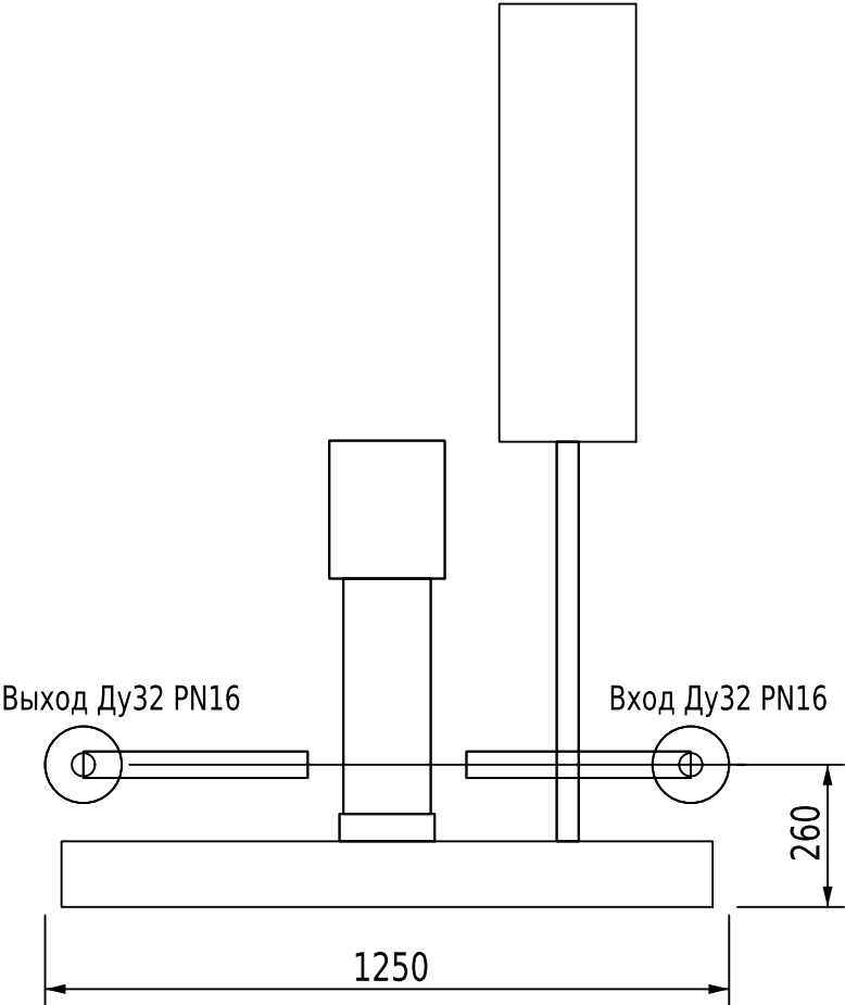
Вид слева
