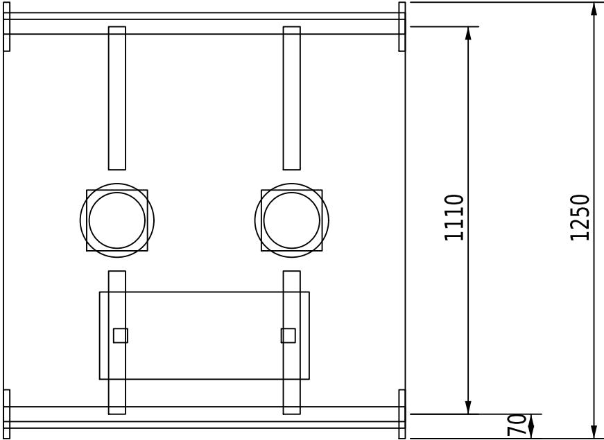
Вид сверху
